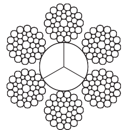
6X36 (14/7+7/7/1) AF SUPERFLEXIBLE
